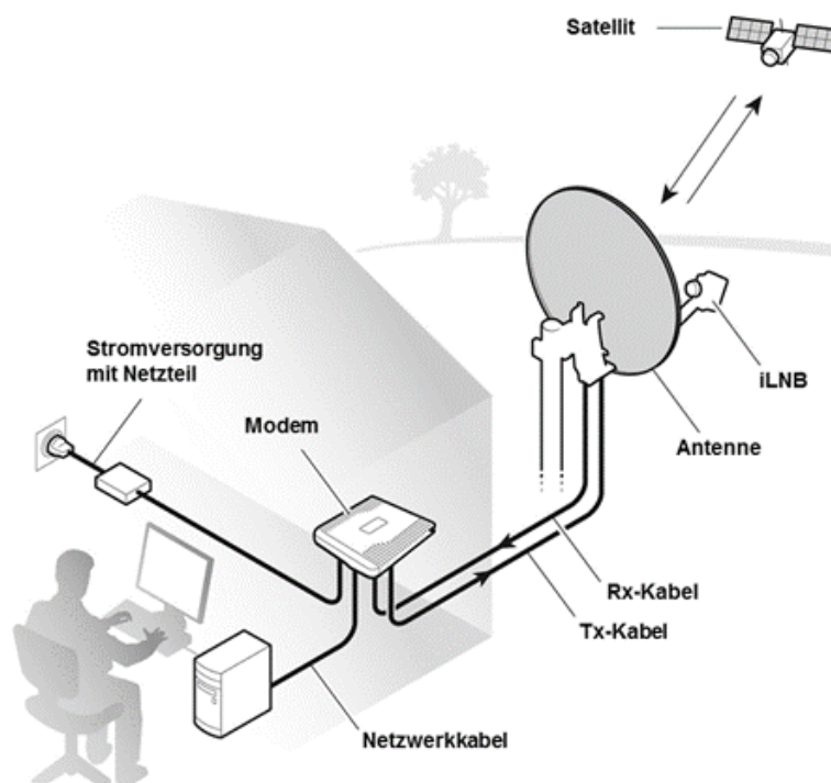
Abbildung 10: SAT-Internetanschluss
